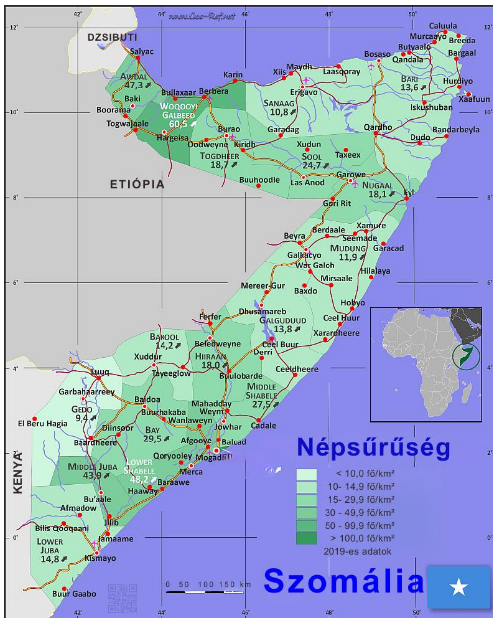
10. ábra: Szomália népsűrűségi térképe 2014-es adatok alapján, saját magyarítással. Forrás: Federal Republic of Somalia 2014.
